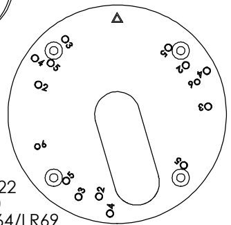
HOLE POSITION DIAGRAM 孔位圖
